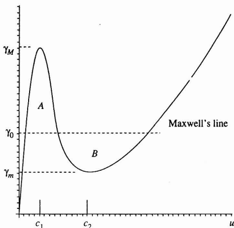
FIG. 1. van der Waals type curve
