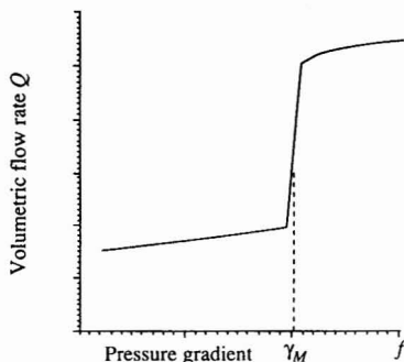
FIG. 5. Spurt
