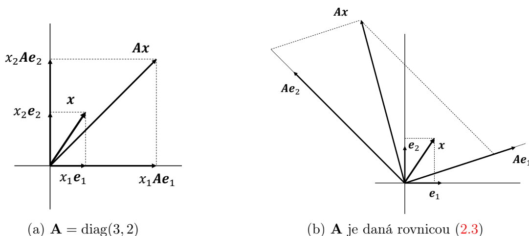
Obr. 2.1: Lineárne zobrazenie \mathbf{A}\mathbf{x} pre \mathbf{x} \in \mathbb{R}^2 .
