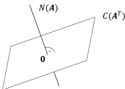
Obr. 3.2: Schematické znázornenie ortogonálnosti \mathcal{N}(\mathbf{A}) a \mathcal{C}(\mathbf{A}^T) .
