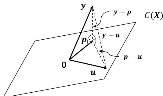
Obr. 7.3: Geometrické znázornenie vety 7.29 a poznámky 7.30. Vektor \mathbf{p} vyjadruje projekciu \mathbf{P}_{\mathbf{X}}\mathbf{y} , prerušované čiary znázorňujú vektory \mathbf{y} - \mathbf{u} , \mathbf{y} - \mathbf{P}_{\mathbf{X}}\mathbf{y} a \mathbf{P}_{\mathbf{X}}\mathbf{y} - \mathbf{u} .
