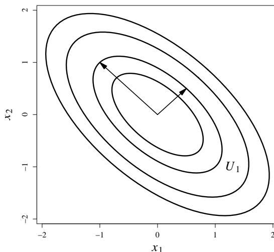
Obr. 10.3: Znáznorenie úrovnových množín U_{1/2} , U_1 , U_2 a U_3 kvadratickej formy zadanej v príklade 10.47. Šípky znázorňujú polosi elipsy U_1 , čiže \mathbf{u}_1/\sqrt{\lambda_1} a \mathbf{u}_2/\sqrt{\lambda_2} .
